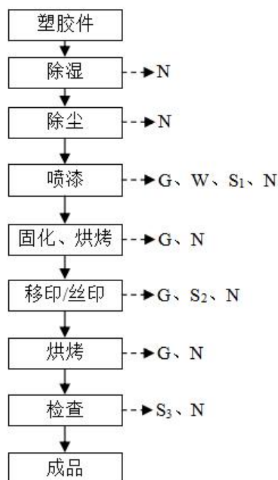
图 3-3 项目塑胶制品生产工艺及产污环节流程图
