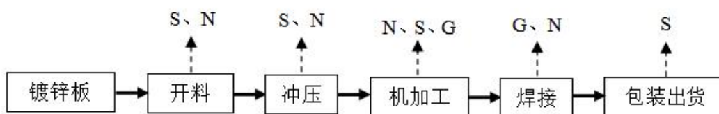
图 3-2 生产工艺及产污环节图
