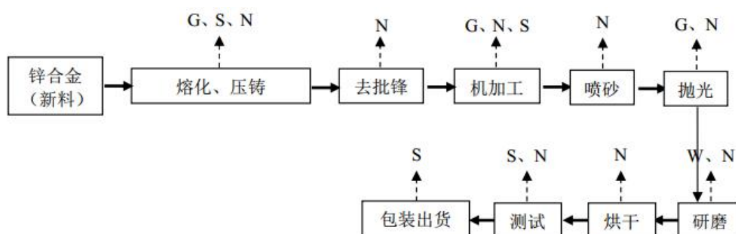
图 3-3 项目五金配件生产工艺及产污环节流程图
